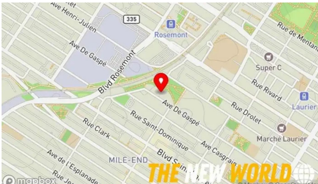
Gologic map
